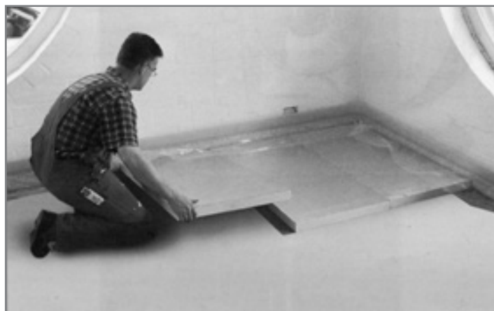
Укладка изоляции PUR
