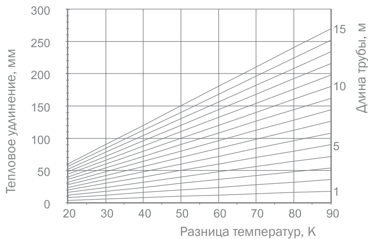
Температурное удлинение для труб РЕ-Хс и РЕ-MDXc TECeFlex
